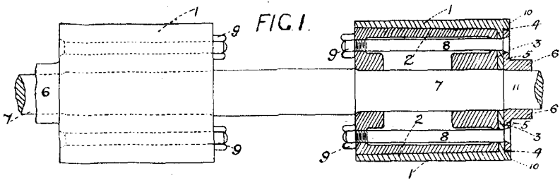
17729 Douglas. Dredge-roller Protector.
